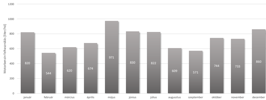
Motorbenzin felhasználásának historikus alakulása
