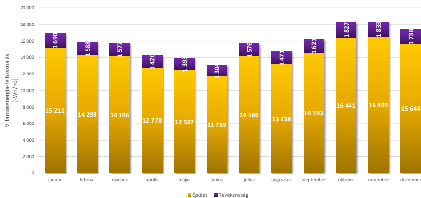
Részterületek villamosenergia felhasználásának historikus alakulása
