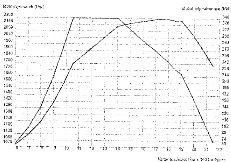
A hajtómotor teljesítmény-nyomaték diagramja
